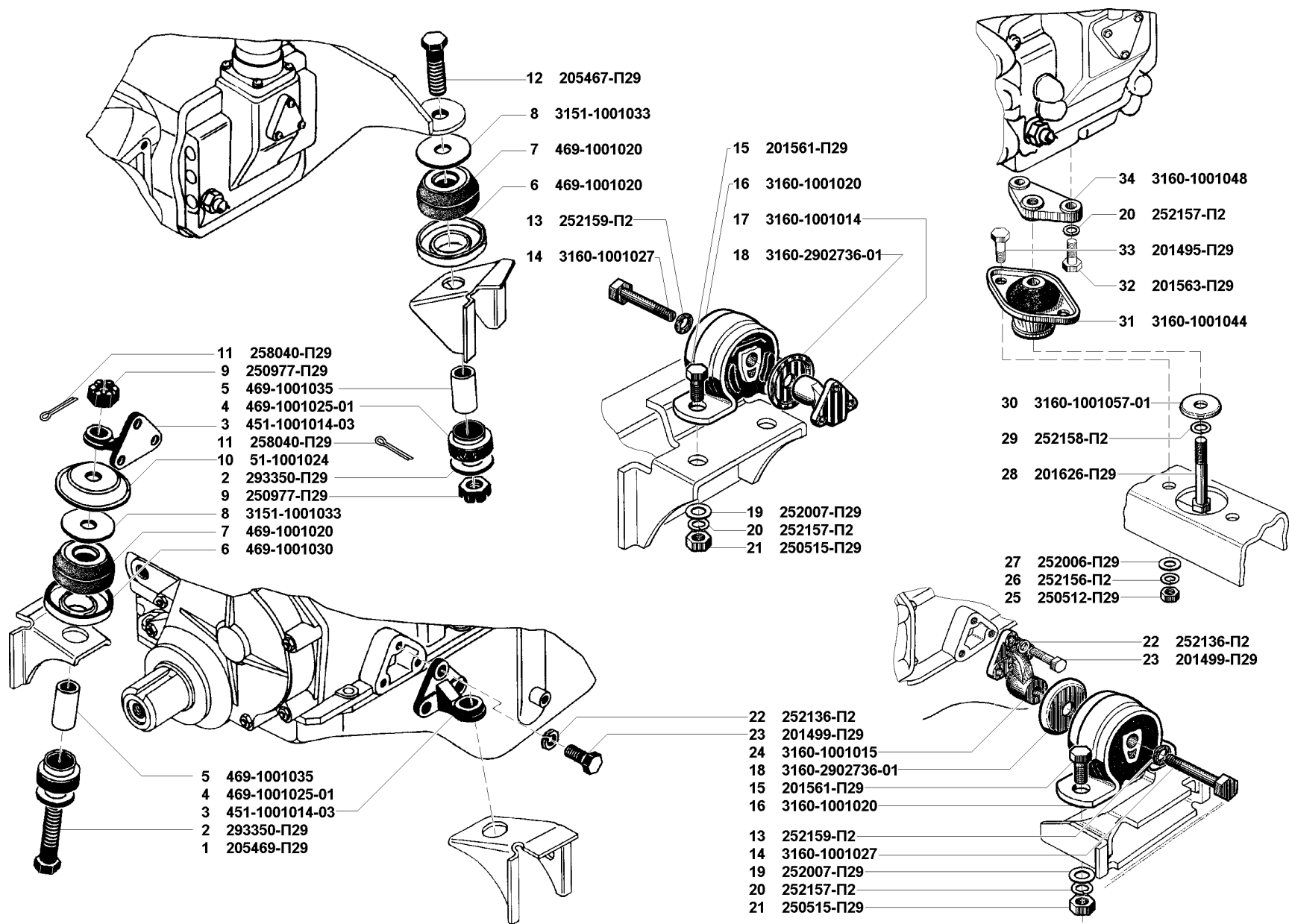
Рис. 4. Подвеска двигателя (1001)
